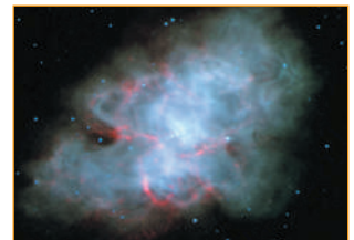
Рис. 3.4. Крабоподібна туманність, яка утворилася після спалаху Надвної у 1054 р.
