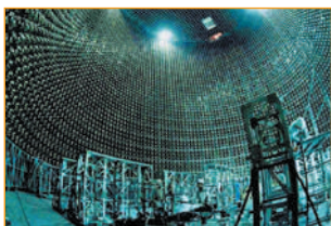
Рис. 2.2. Підземний детектор нейтрино
