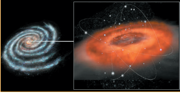
Рис. 2.4. Надмасивна чорна діра Стрілець А*
