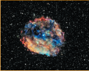
Рис. 3.7. Туманність Кассіопеї
