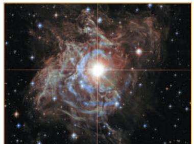
Рис. 2.3. Цефеїди
