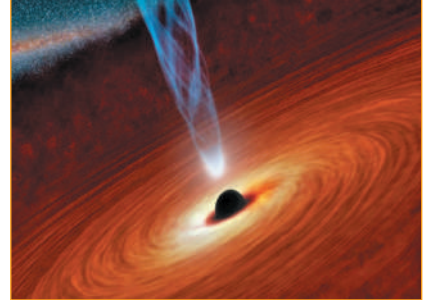
Рис. 2.5. Комп'ютерна модель чорної діри в центрі Галактики
