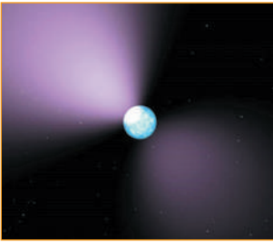
Рис. 3.7. Художнє зображення пульсара
