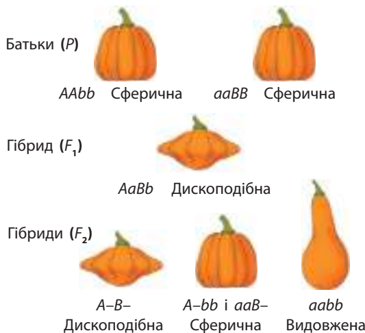
Мал. 64.2. Комплементарна взаємодія генів
