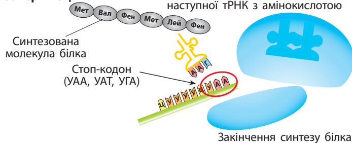
Мал. 43.1. Схема трансляції
