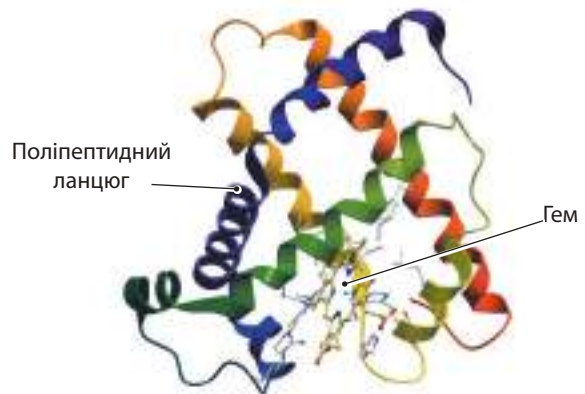
Мал. 30.2. Молекула міоглобіну людини
