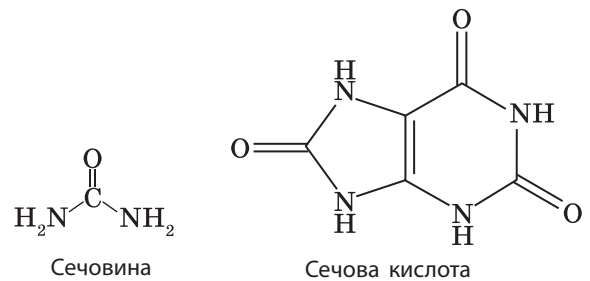
Мал. 41.3. Нітрогеновмісні кінцеві продукти катаболізму
