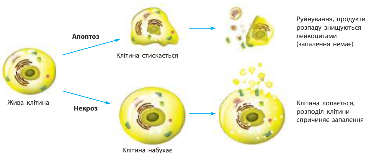
Мал. 85.1. Процеси, що відбуваються під час апоптозу та некрозу
