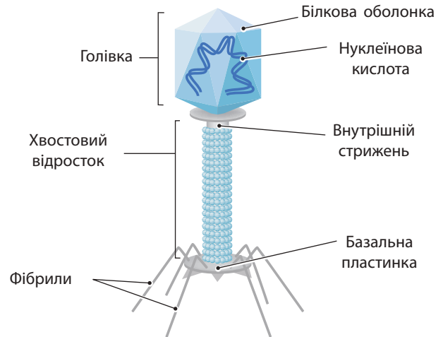
Мал. 72.3. Будова бактеріофага
