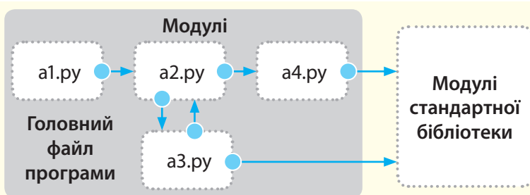
Рис. 1. Варіант структури проекту мовою Python
