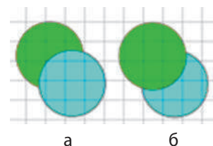
Рис. 1. Перекриття об'єктів
