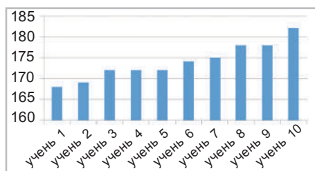
Рис. 2. Гістограма зросту учнів (за абсолютним значенням)
