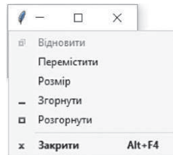
Рис. 4. Системне меню
