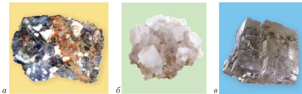
Рис. 55. Мінерали: а — сільвініт; б — кристалічний натрій хлорид; в — галіт
