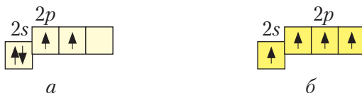
Рис. 15. Графічні електронні формули атома Карбону в основному (а) і збудженому (б) станах
