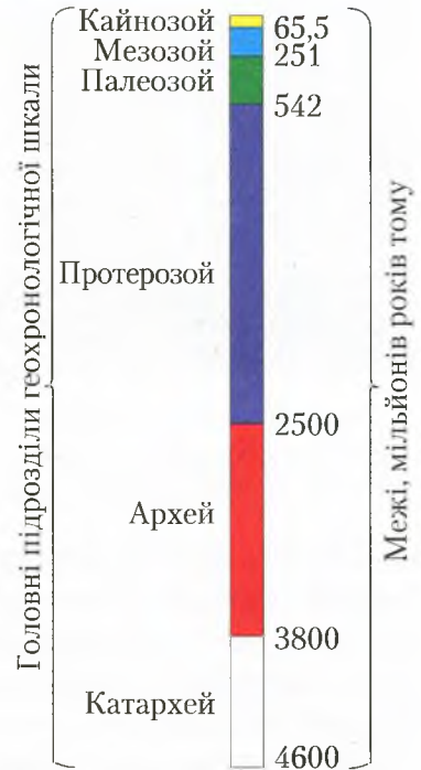
Рис. 62.2. Геохронологічна шкала
