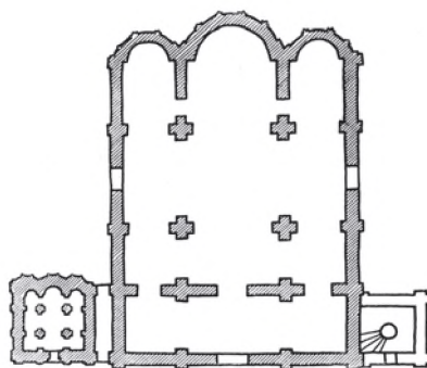
Успенський собор Києво-Печерської лаври (реконструкція і план)
