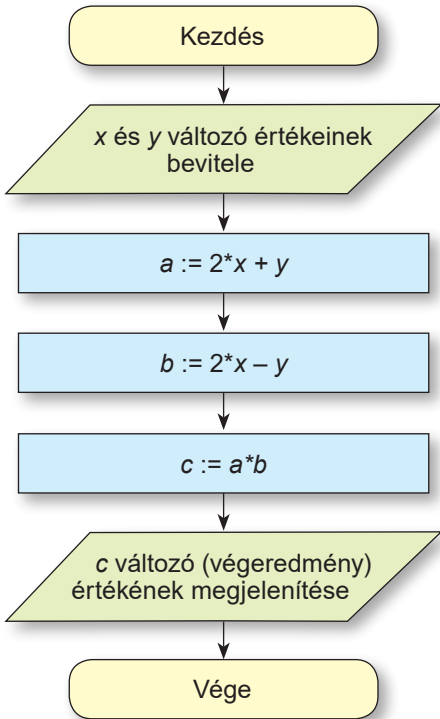
4.5. ábra. Az (2*x + y)*(2*x - y) kifejezés értékének kiszámításához használt algoritmus blokkdiagramja
