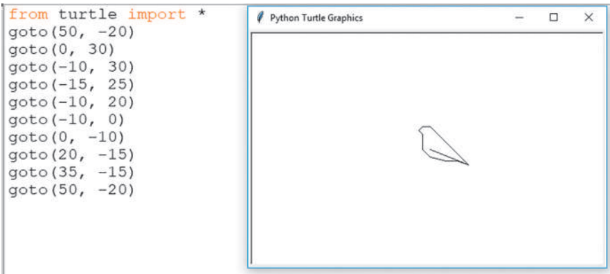
4.14. bra. Program egy s v lt  lerajzolas hoz Python -ban
