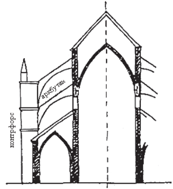
Структура готичного собору у поперечному розрізі
