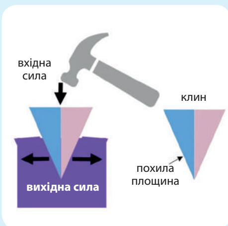
Мал. 104. Дія клина
