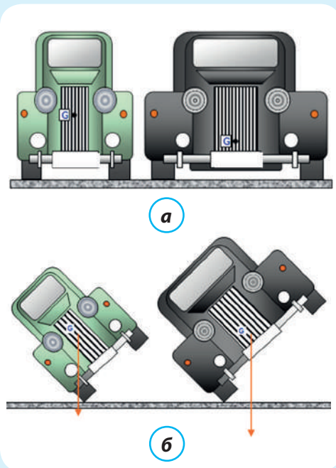
Мал. 86. а — положення центру ваги тіла (G); б — зміна положення центру ваги тіла
