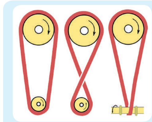
Мал. 121. Розташування шківів пасової передачі
