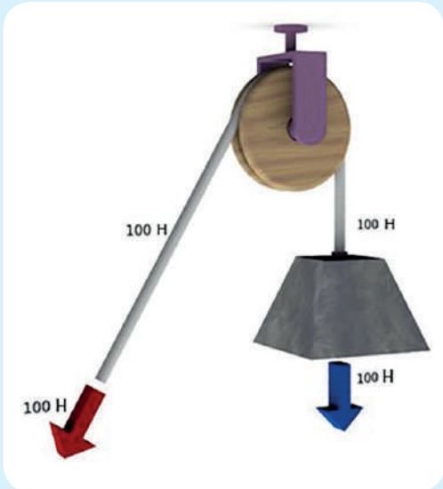
Мал. 93. Нерухомий блок (шків)
