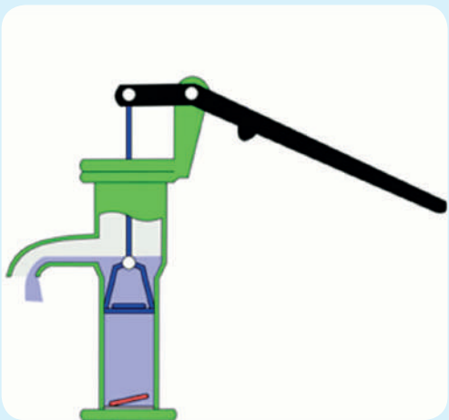
Мал. 28. Будова поршневого насоса
