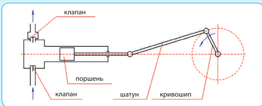
Мал. 27. Будова нагнітального (поршневого) насоса
