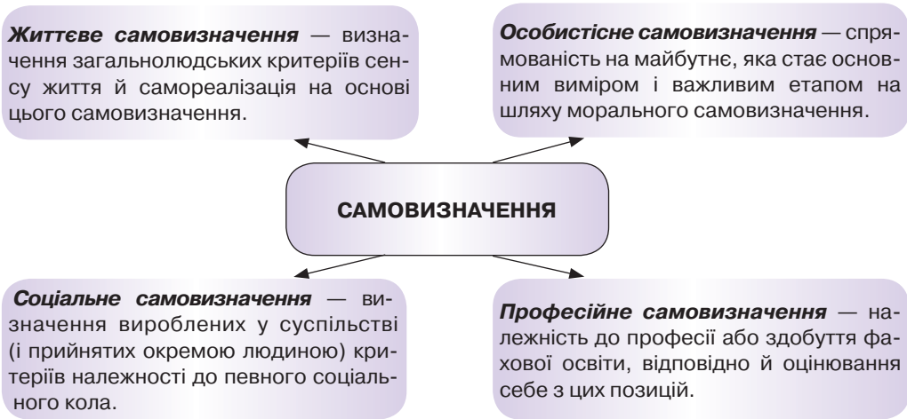
Схема 5
